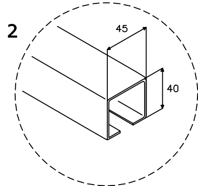
C-profiel bovenrail Cod. 003
