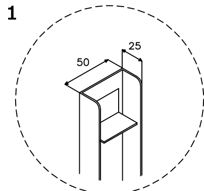
Stijl met onder- steuningslip Cod. 008
